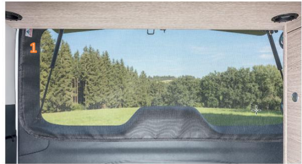
Die Klettverschlussbefestigung des FLYOUT dient alternativ auch zur Befestigung des ISOLITE für das Heckklappenfenster.
